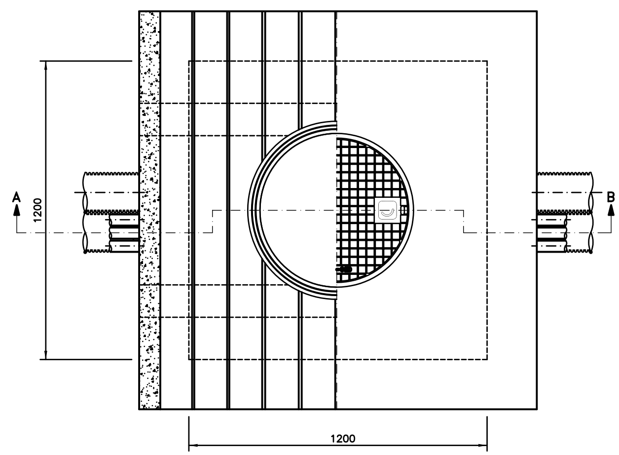
PLANTA
