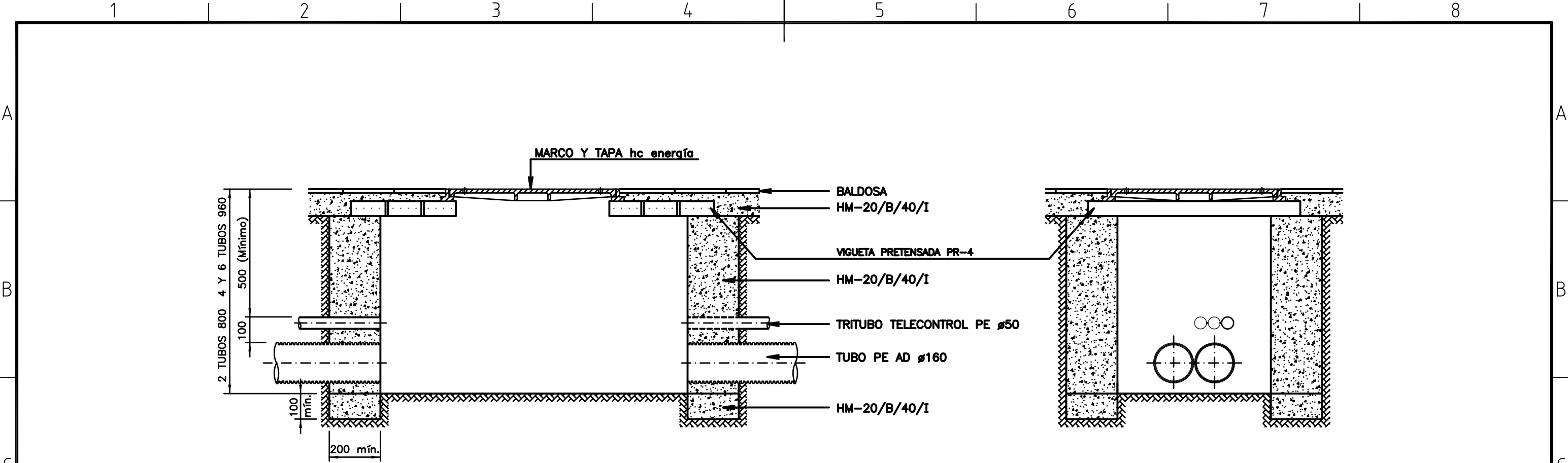
SECCION A-B
