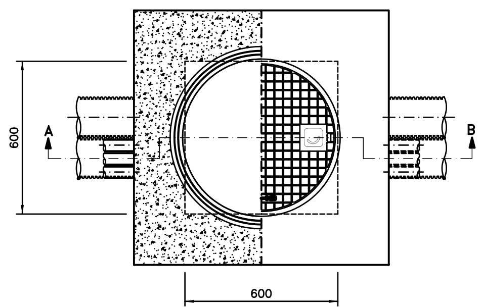
PLANTA
