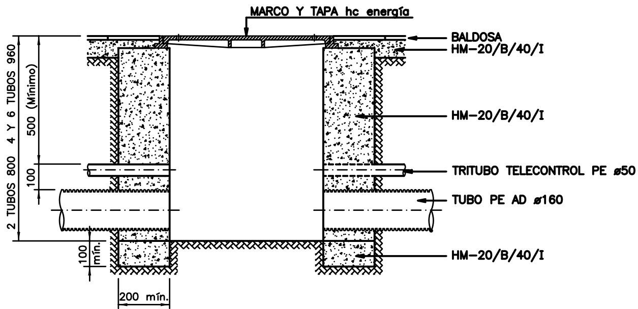
SECCION A-B
