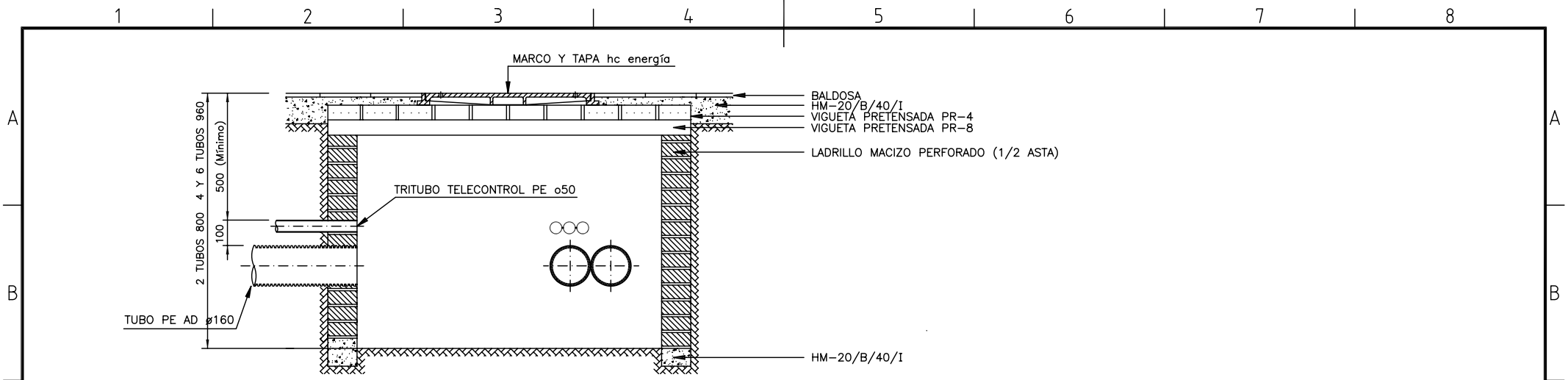
SECCION A-B
