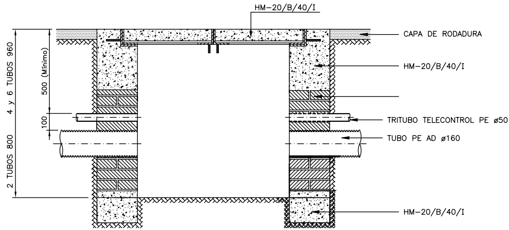
SECCION A-B
