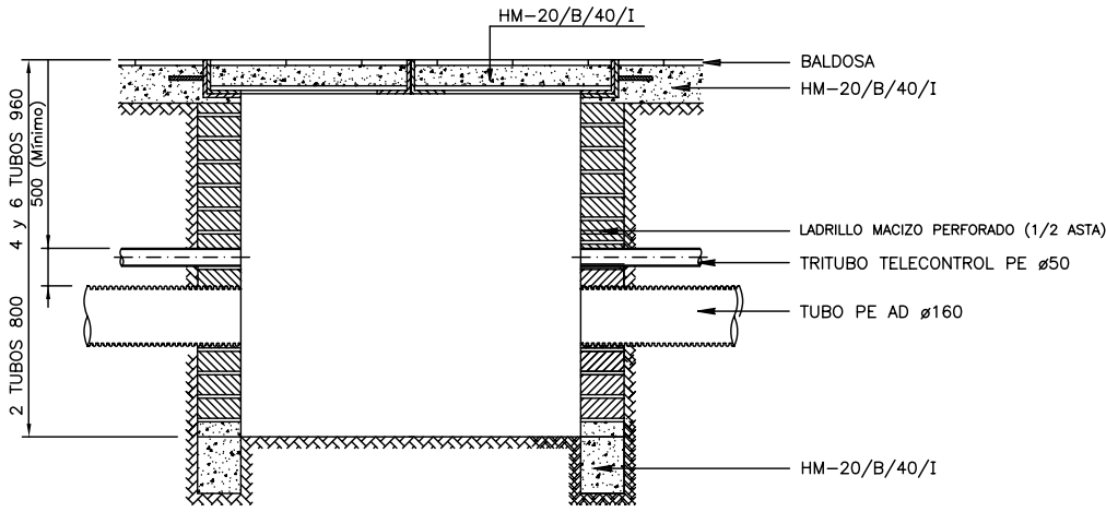
SECCION A-B
