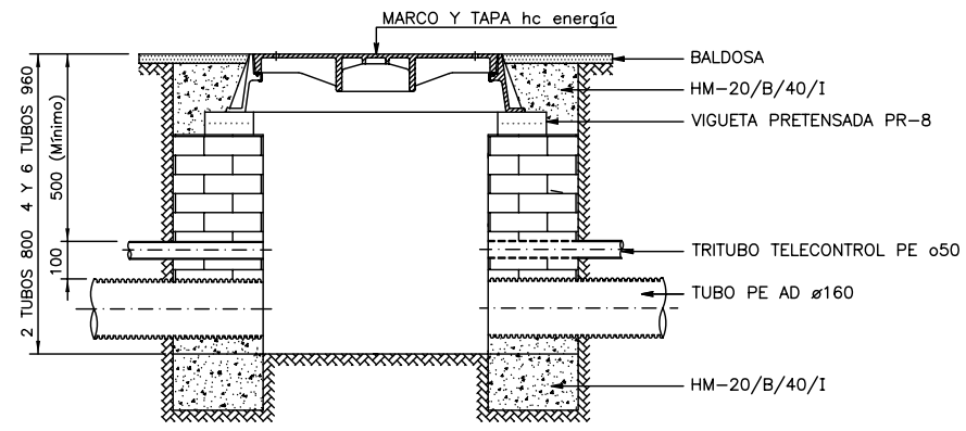
SECCION A-B
