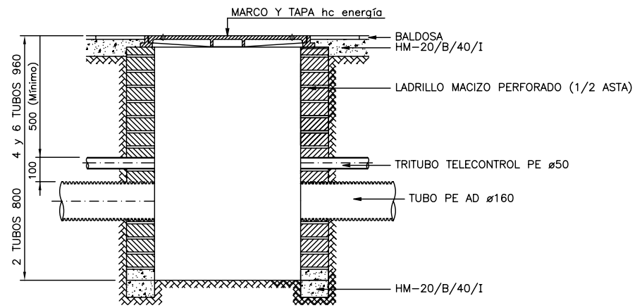
SECCION A-B
